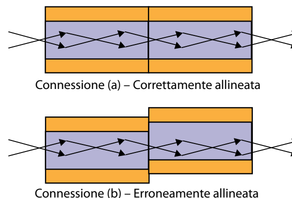
Figura 15 – Misurare le due connessioni rappresentate in condizioni di "underfilled launch" può non mettere in evidenza problemi di disallineamento nel cavo ottico.
