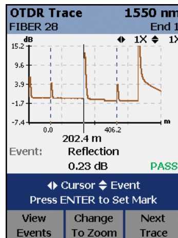
Figura 23 – TRACE Anzeige eines DTX Compact OTDRs (850nm)
