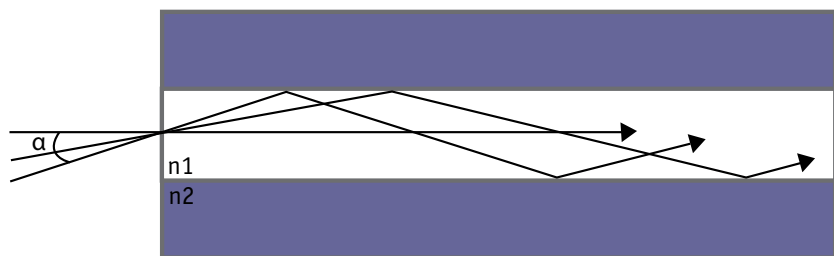
Figura 8 - La fibra ottica accetta tutta la luce che entra con un'angolazione massima indicata dall'Apertura Numerica. La luce si riflette sulla superficie di separazione tra core e cladding e si propaga secondo percorsi differenti. Questi percorsi sono chiamati modi. La fibra ottica multimodale guida la luce attraverso molti modi, cioè molti percorsi. La luce che entra secondo angoli più ampi segue percorsi più lunghi. Ciò rappresenta i modi di propagazione di ordine superiore.
