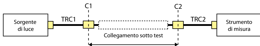
Figura A2-2 Misura della perdita ottica con il metodo two-jumper – La 'differenza' tra il livello di energia di riferimento e il valore misurato rappresenta la perdita nel link sotto test, la perdita nella connessione C2 e la differenza tra la perdita in CR1 e quella relativa a C1. Questa differenza può variare; l'attenuazione totale relativa a C1 non è compresa nel risultato del test.
