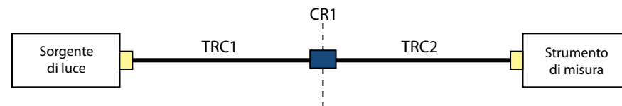
Figura A2-3 - Il metodo 'one-jumper modificato' utilizza esattamente la stessa procedura di impostazione del riferimento del metodo two-jumper. Da sottolineare che le TRC sono bretelle ibride terminate ad una estremità con un connettore compatibile con l'apparecchiatura di test e all'altra con un connettore dello stesso tipo di quello utilizzato dal link sotto test. La figura evidenzia i diversi tipi di connettori utilizzando colori diversi.
