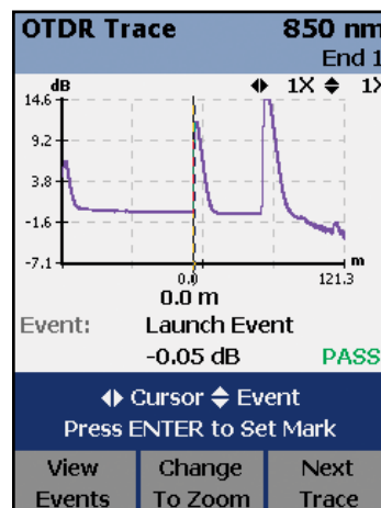
Figura 24 – TRACE Anzeige eines DTX Compact OTDRs (1300nm)
