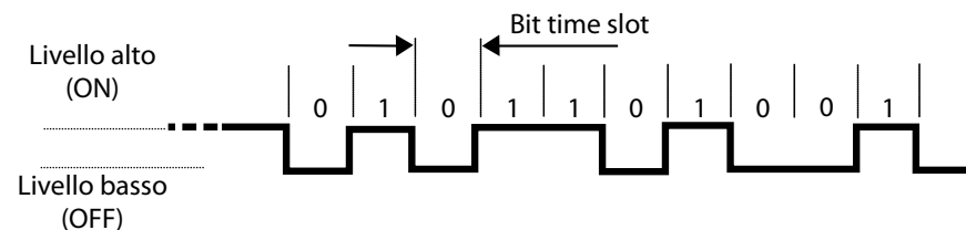
Figura 4 - Un tipico treno di impulsi che rappresenta i dati digitali
