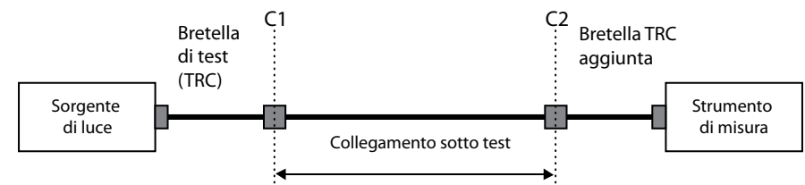
Figura 14 – Collegamento della sorgente di luce 'Light Source' e dello strumento 'Power Meter' per la misura dell'attenuazione ottica
