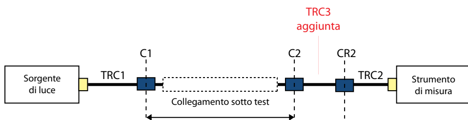
Figura A2-4 Il metodo 'One-jumper modificato' per la misura della perdita ottica – La 'differenza' tra il livello di potenza di riferimento e il valore misurato rappresenta la perdita del link sotto test, la perdita delle connessioni C1 e C2, la perdita della fibra della bretella TRC3 e la differenza tra le perdite associate alle connessioni CR1 e CR2 (due connessioni di riferimento).
