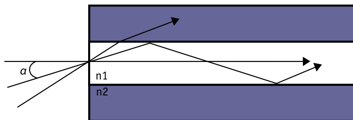
Figura 3 - Apertura numerica e riflessione totale: la luce che entra nella fibra con un angolo viaggia nel core.
