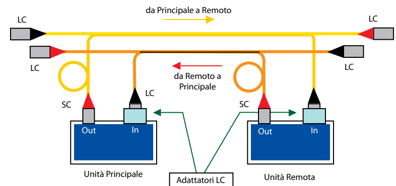
Figura 18e – Rappresentazione schematica dell'impostazione del riferimento con TRC duplex per un link da testare che termina con connettori LC. L'anello vicino al connettore rosso indica il posizionamento del mandrino (per fibra multimodale).
