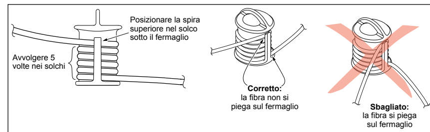
Figura 16 – Come avvolgere correttamente la bretella ottica di test attorno al mandrino
