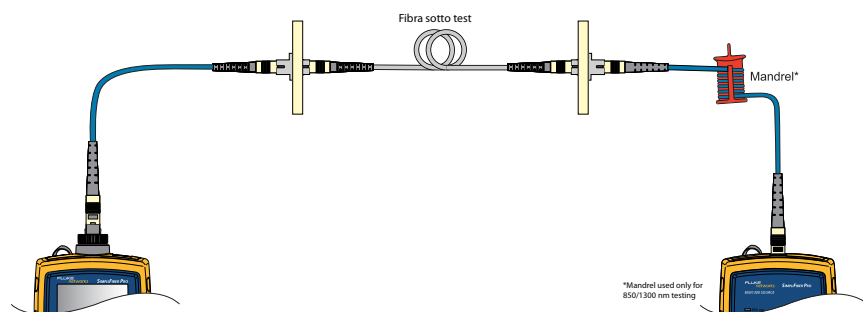
Figura 17 – L'esecuzione di un test LSPM
