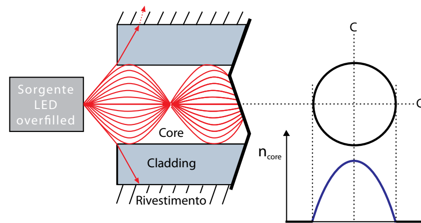
Figura 10 - Fibra multimodale graded index. L'indice di rifrazione del core non è costante all'interno del core. È più alto al centro e gradualmente diminuisce progredendo verso il confine con il cladding. Questa struttura crea percorsi della luce (modi) con andamento a serpentina come illustrato nella parte sinistra della figura. I modi di ordine inferiore (al centro del core) viaggiano a velocità più bassa, mentre i modi più esterni che compiono le distanze maggiori viaggiano a velocità media più alta. Le fibre multimodali graded index quindi sono caratterizzate da una larghezza di banda maggiore.
