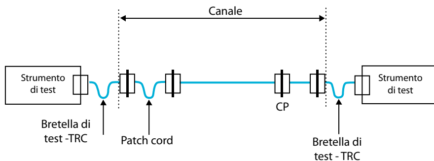
Figura 12 – Le connessioni alle estremità in Fig 12 non sono comprese nelle specifiche di canale. Sostituendo le bretelle di apparato con delle Test Reference Cords (TRCs) per misurare l'attenuazione complessiva di canale e la lunghezza, l'errore nella misura di perdita è rappresentato dalla differenza in lunghezza tra una TRC e la somma delle due bretelle di apparato utilizzate per completare il canale. 1 m di bretella rappresenta 0.0035 dB.
