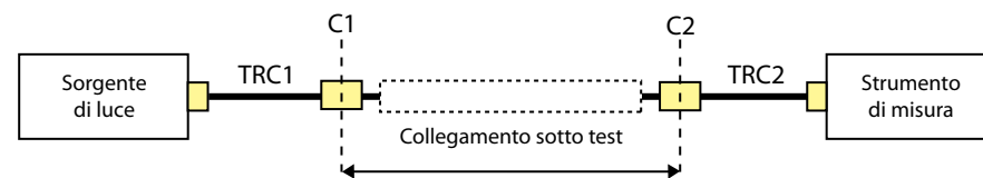
Figura A2-6 - Misura della perdita ottica con il metodo 'Three-jumper' – La 'differenza' tra il livello di potenza di riferimento e il valore misurato rappresenta la perdita del link sotto test, la differenza tra la perdita della connessione di riferimento CR1 e C1 e la differenza tra la perdita della connessione di riferimento CR2 e C2. La perdita effettiva nelle connessioni C1 e C2 non è inclusa nel risultato della misura.
