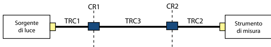
Figura A2-5 - Metodo 'Three-jumper' – Nella misura del riferimento per il test è compresa la perdita nella connessione tra la bretella di test 1 (TRC1) e la sorgente di luce, la perdita nelle bretelle TRC1, TRC2 e TRC3, la perdita nelle connessioni di riferimento CR1, CR2 e la perdita nella connessione tra TRC2 e lo strumento di misura dell'energia luminosa.
