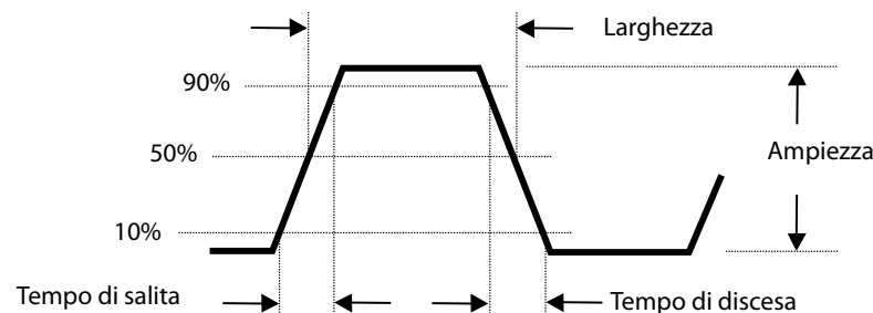
Figura 5 - Analisi di un impulso
