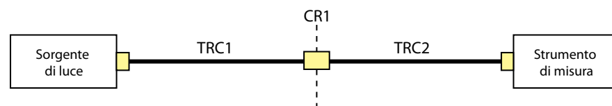
Figura A2-1 Metodo a due bretelle ‘two-jumper’ – Nella misura del riferimento per il test è compresa la perdita nella connessione tra la bretella di test 1 (TRC1) e la sorgente di luce, la perdita nella bretella TRC1, la perdita nella connessione CR1, la perdita nella bretella TRC2 e la perdita nella connessione tra TRC2 e lo strumento di misura dell’energia luminosa..
