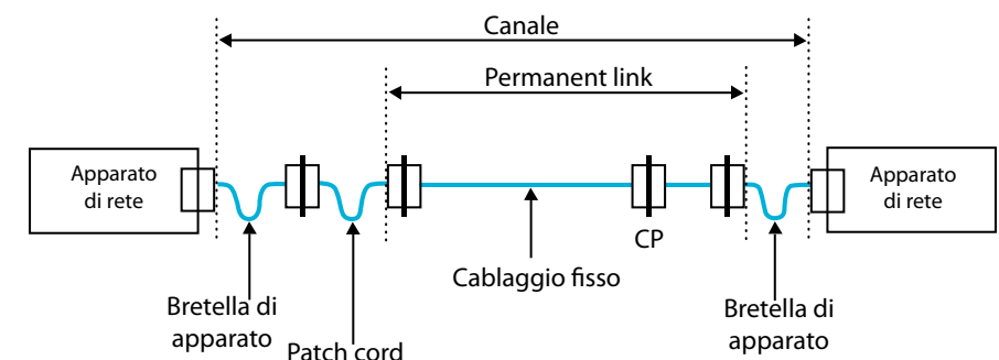
Figura 11 – Il canale è il collegamento completo dal trasmettitore al ricevitore. Il cablaggio fisso – una parte di tutto il canale – è chiamato permanent link. La figura mostra il modello generale di un cablaggio orizzontale che contiene anche connessioni opzionali come il CP (Consolidation Point).
